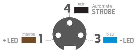
VUE DE FACE DU CONNECTEUR DU PRODUIT
